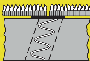
Forma 3 G Połączenie w zygzak, podklejone folią, do szlifowania wykończeniowego pasami szerokimi na podłożu płóciennym, gwarantującego najwyższą jakość powierzchni.
